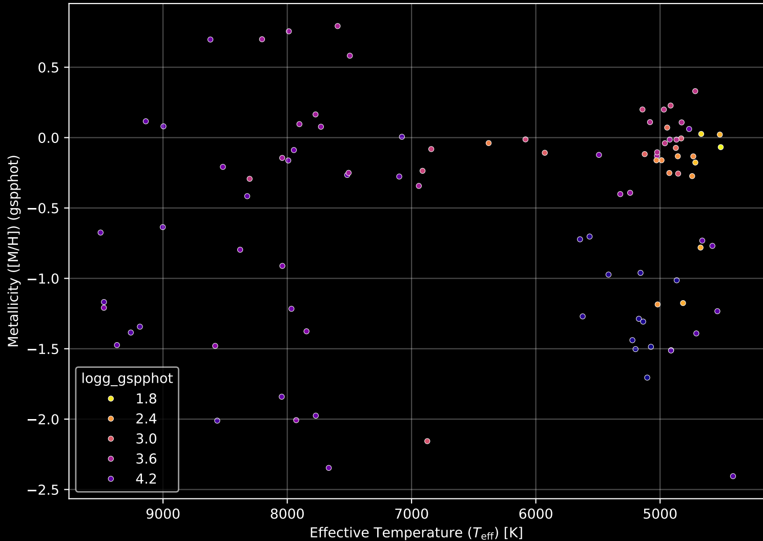
Gaia Cluster: [FSR_0344] Stellar Population Parameters (n= 96)
