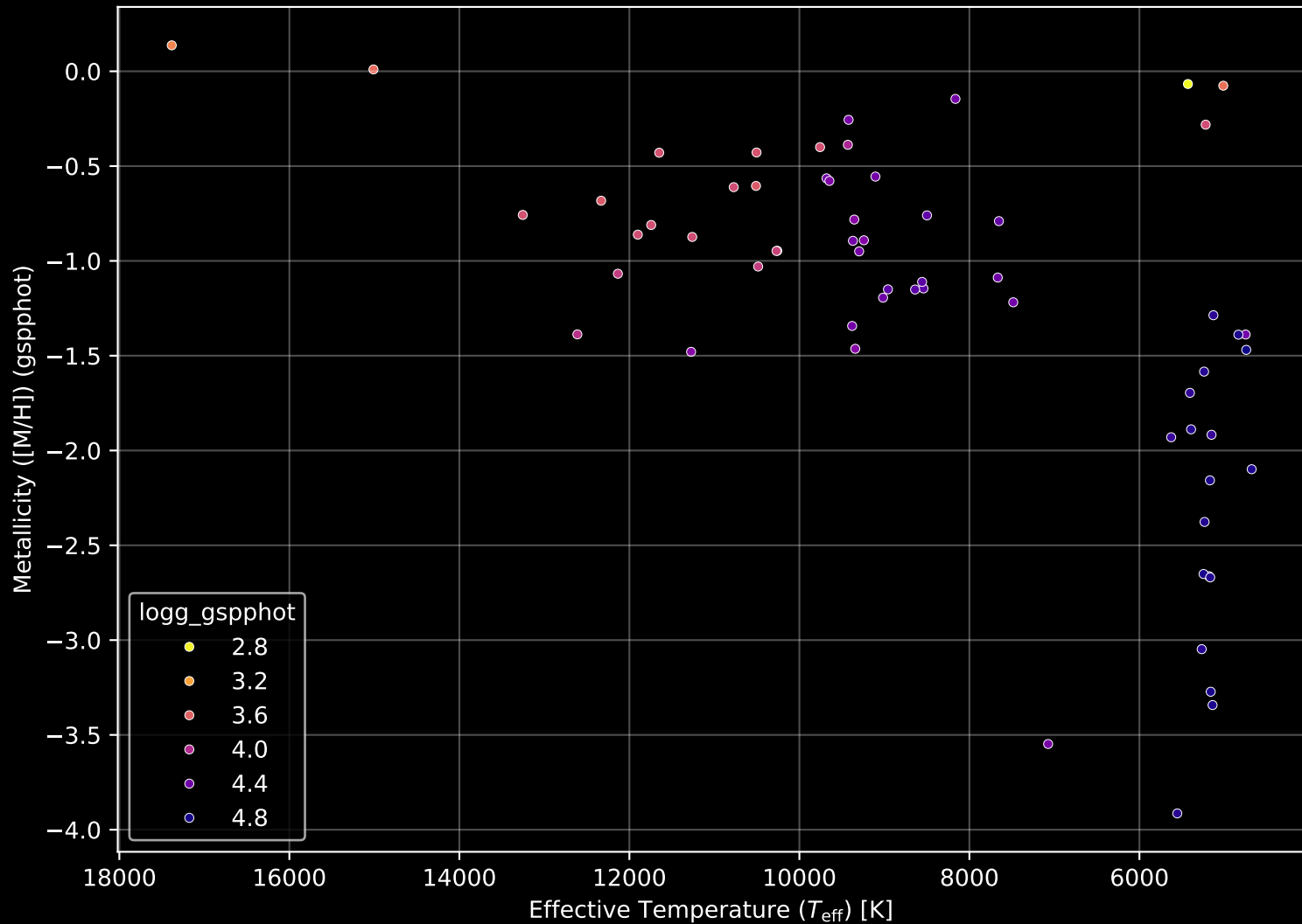
Gaia Cluster: [FSR_0357] Stellar Population Parameters (n= 62)
