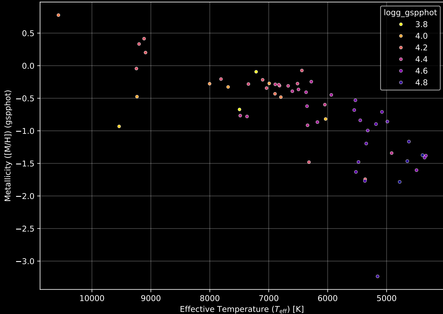
Gaia Cluster: [FSR_0384] Stellar Population Parameters (n= 58)
