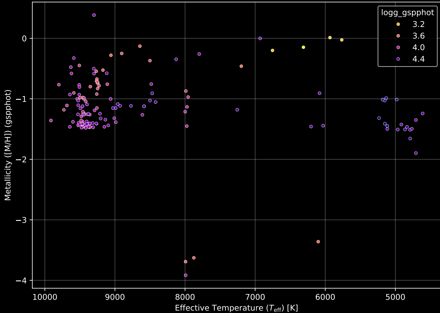
Gaia Cluster: [FSR_0442] Stellar Population Parameters (n= 145)
