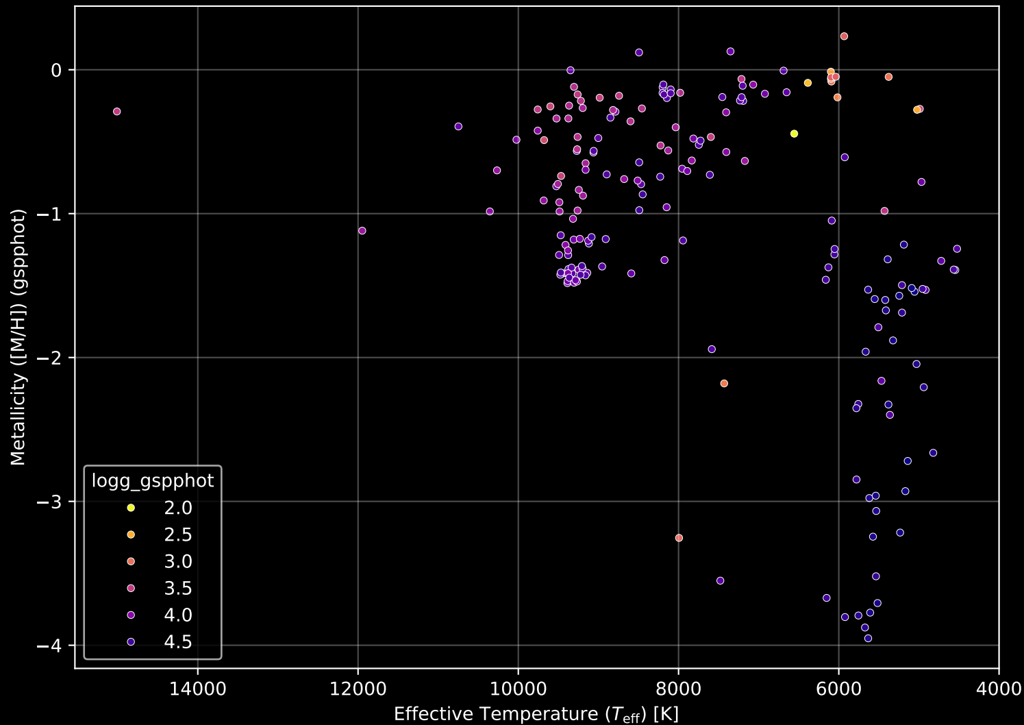
Gaia Cluster: [FSR_0494] Stellar Population Parameters (n= 191)
