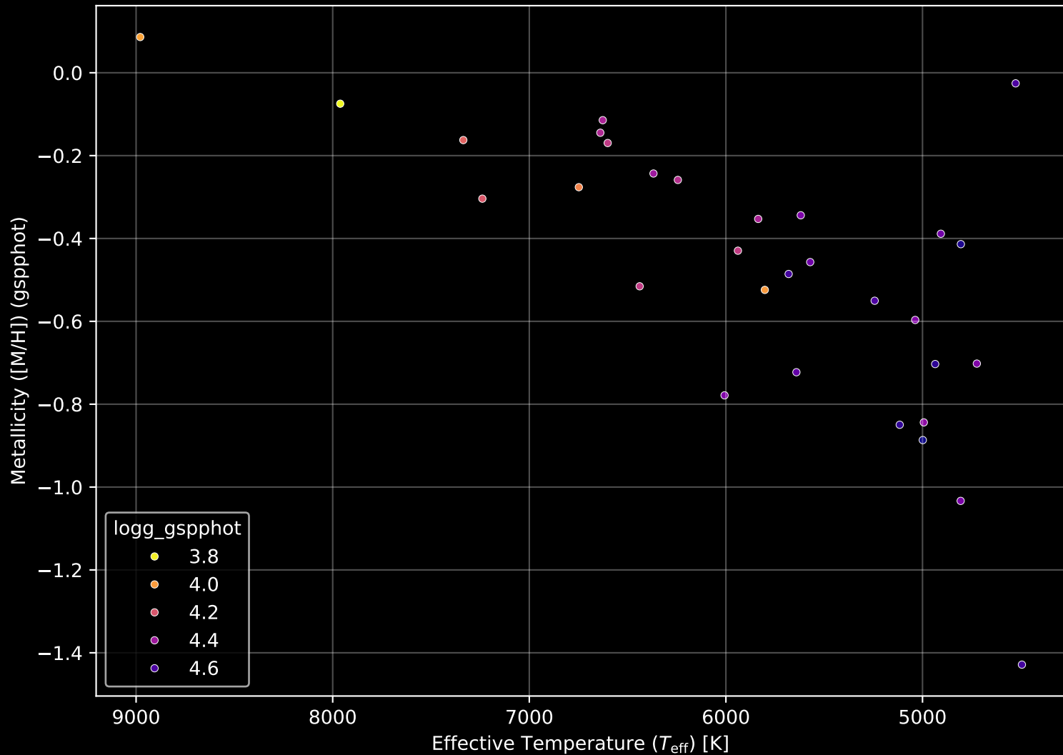
Gaia Cluster: [FSR_0667] Stellar Population Parameters (n= 31)
