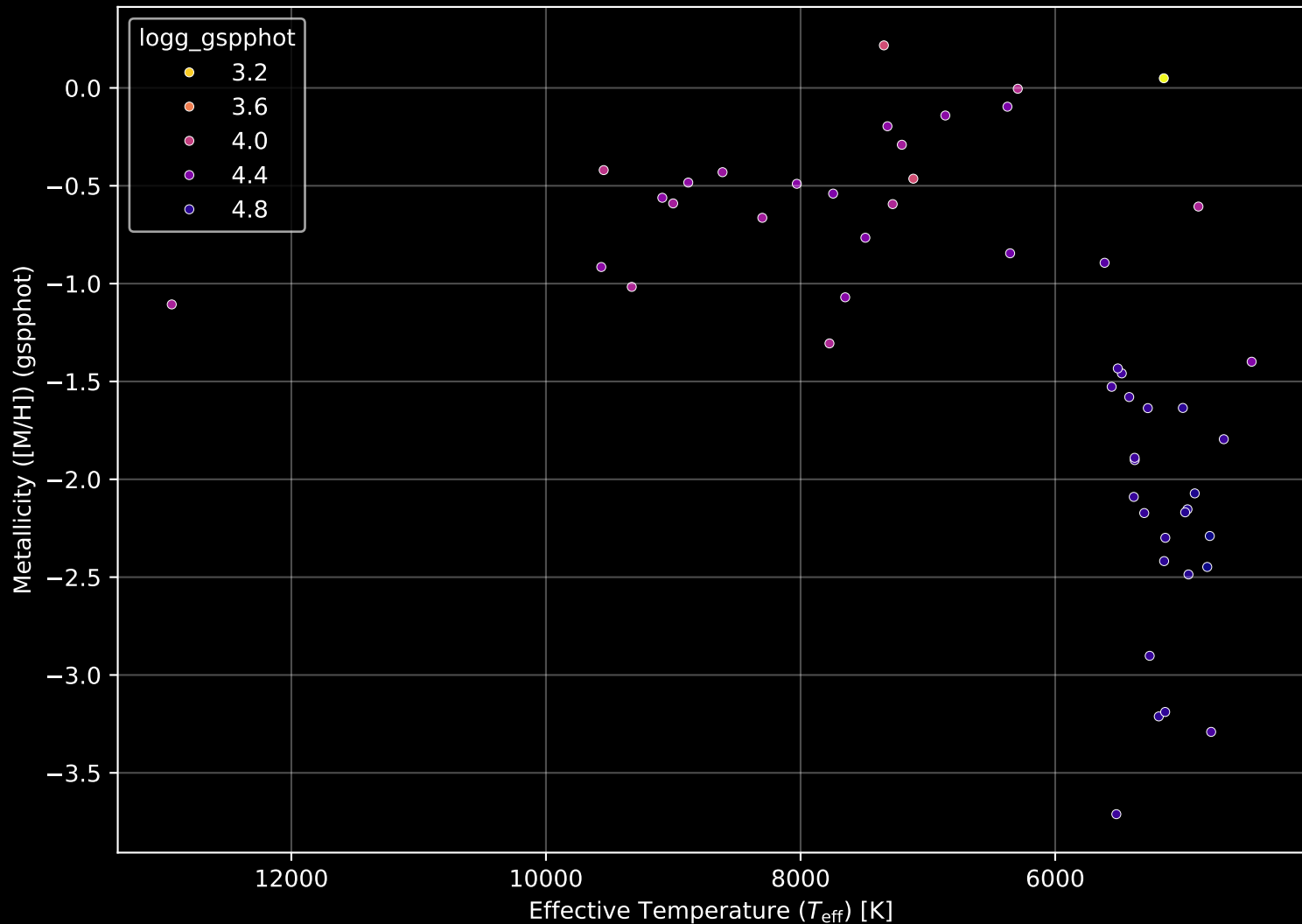
Gaia Cluster: [FSR_0683] Stellar Population Parameters (n= 51)
