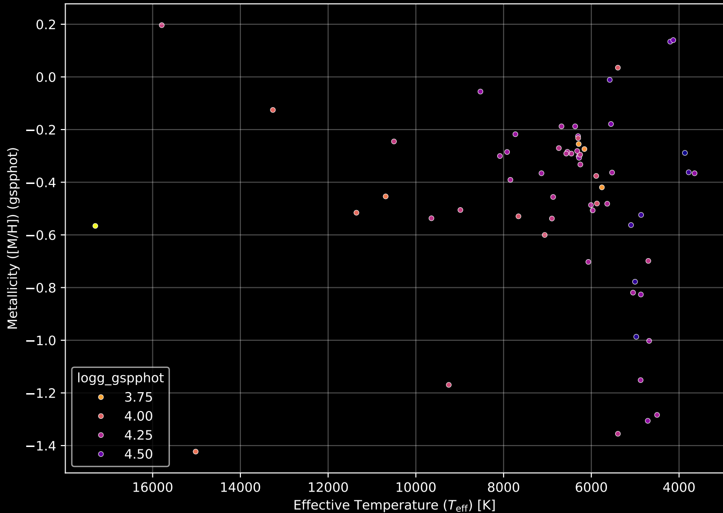
Gaia Cluster: [FSR_0686] Stellar Population Parameters (n= 63)
