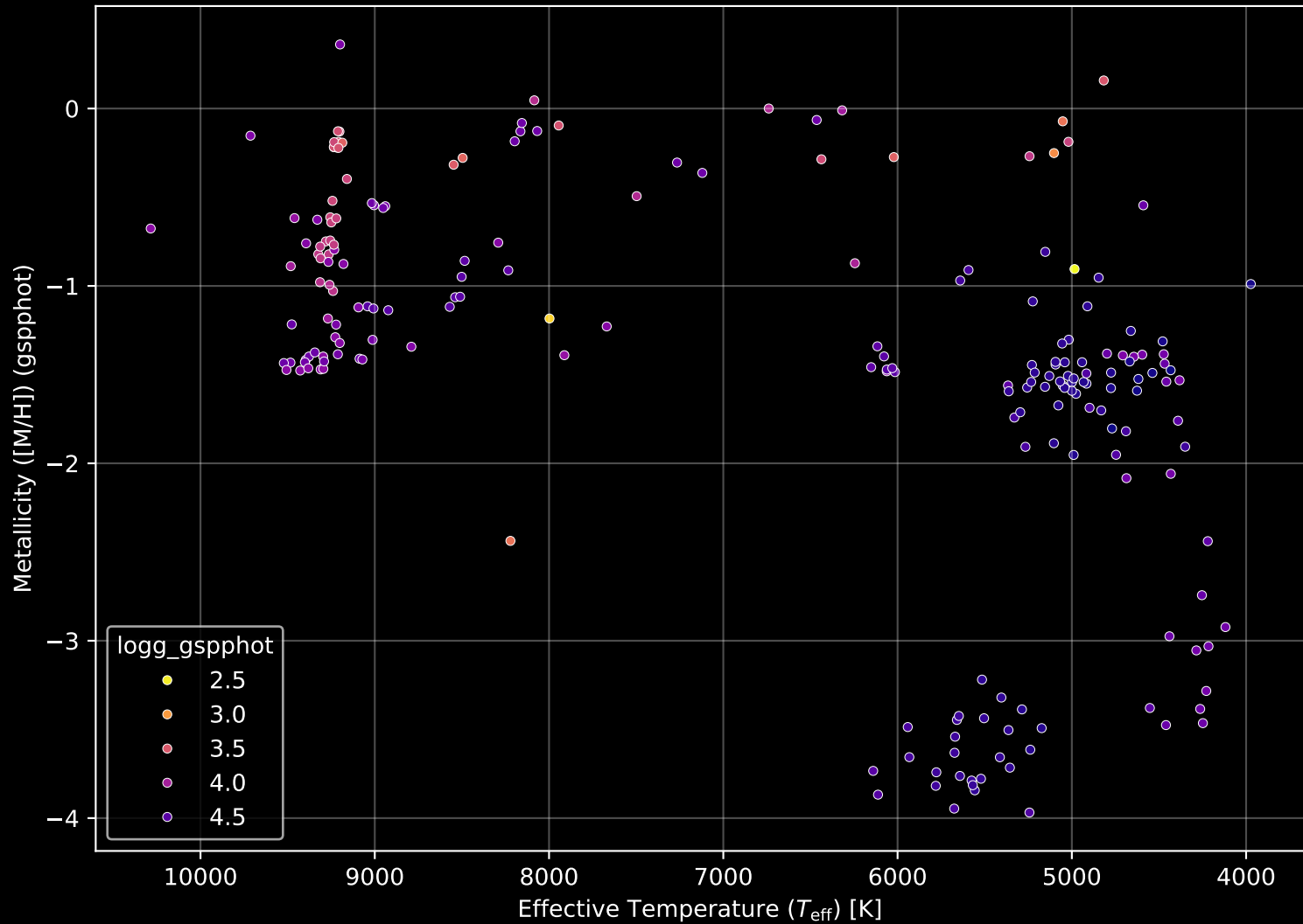
Gaia Cluster: [FSR_0893] Stellar Population Parameters (n= 208)
