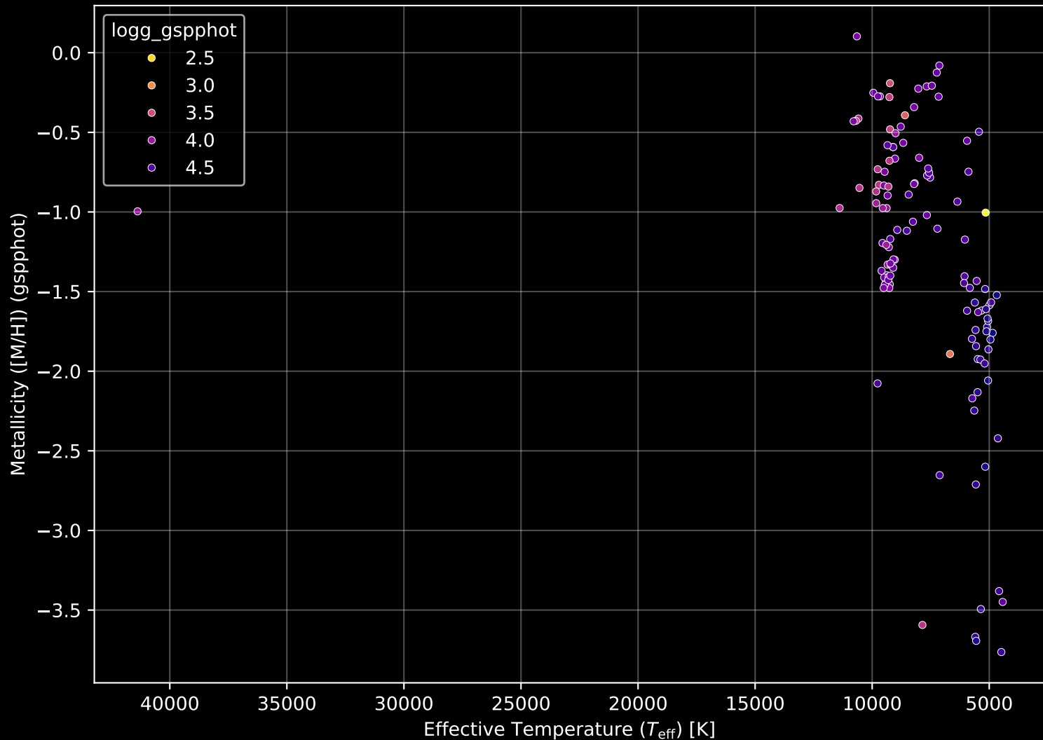
Gaia Cluster: [FSR_0904] Stellar Population Parameters (n= 123)
