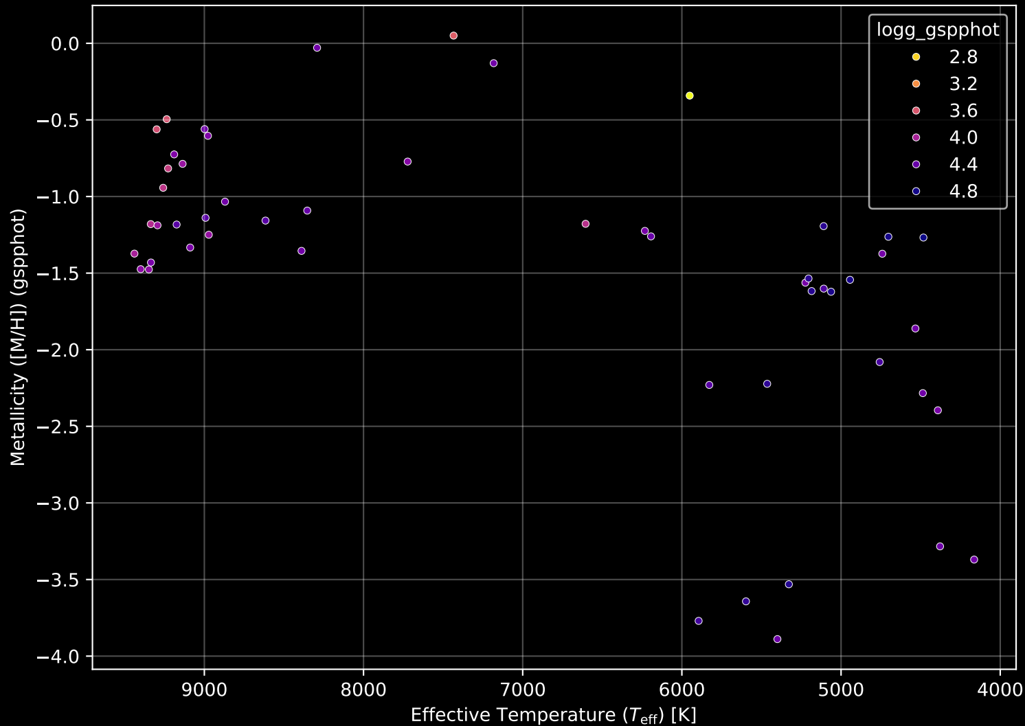
Gaia Cluster: [FSR_0923] Stellar Population Parameters (n= 52)
