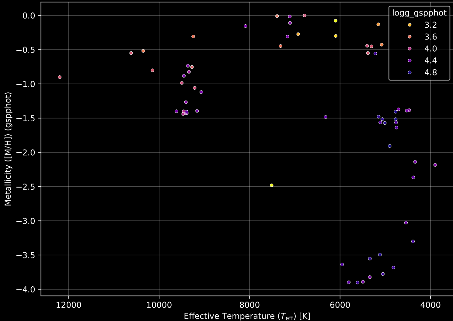
Gaia Cluster: [FSR 0932] Stellar Population Parameters (n= 65)
