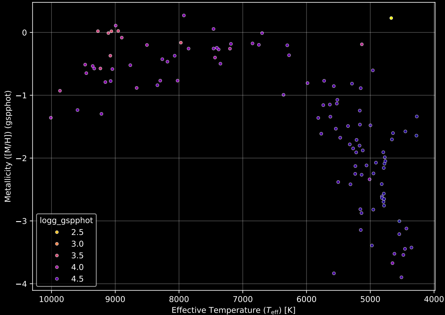
Gaia Cluster: [FSR_0935] Stellar Population Parameters (n= 113)
