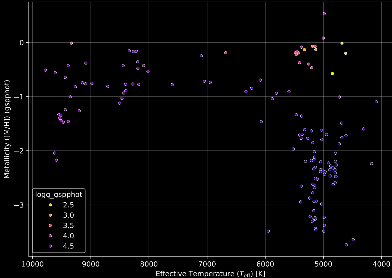
Gaia Cluster: [FSR_0975] Stellar Population Parameters (n= 142)
