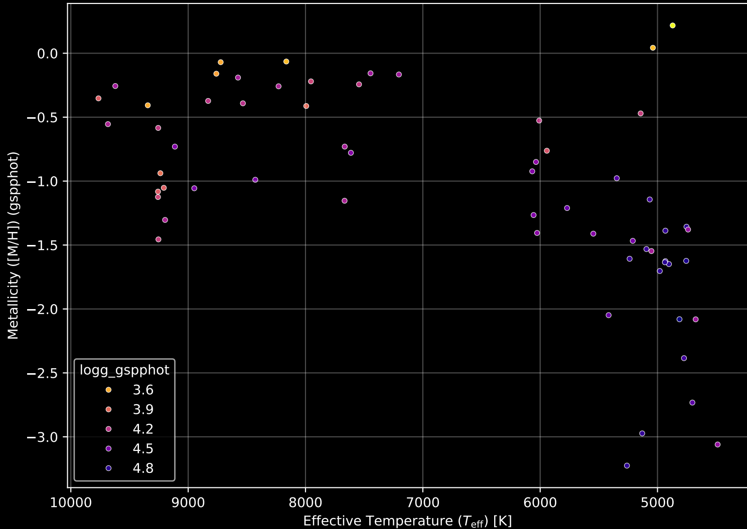
Gaia Cluster: [FSR_1051] Stellar Population Parameters (n= 62)
