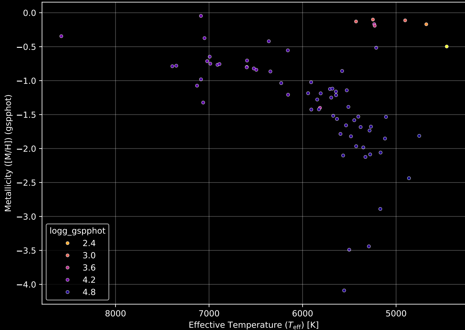
Gaia Cluster: [FSR_1113] Stellar Population Parameters (n= 70)
