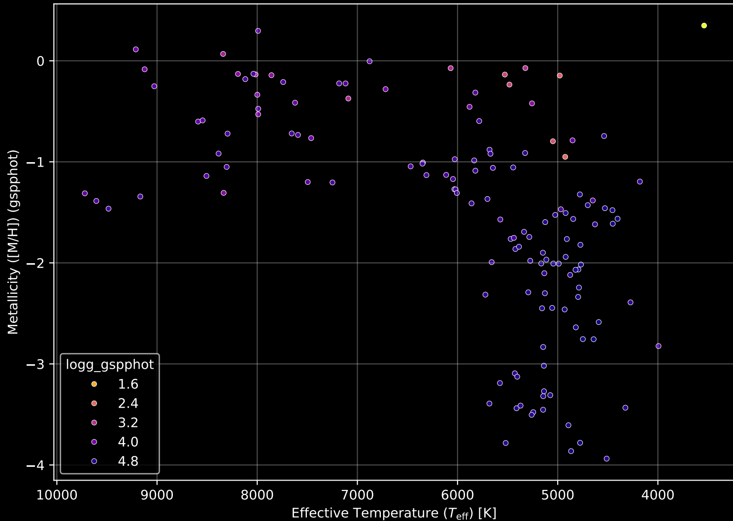
Gaia Cluster: [FSR_1163] Stellar Population Parameters (n= 139)
