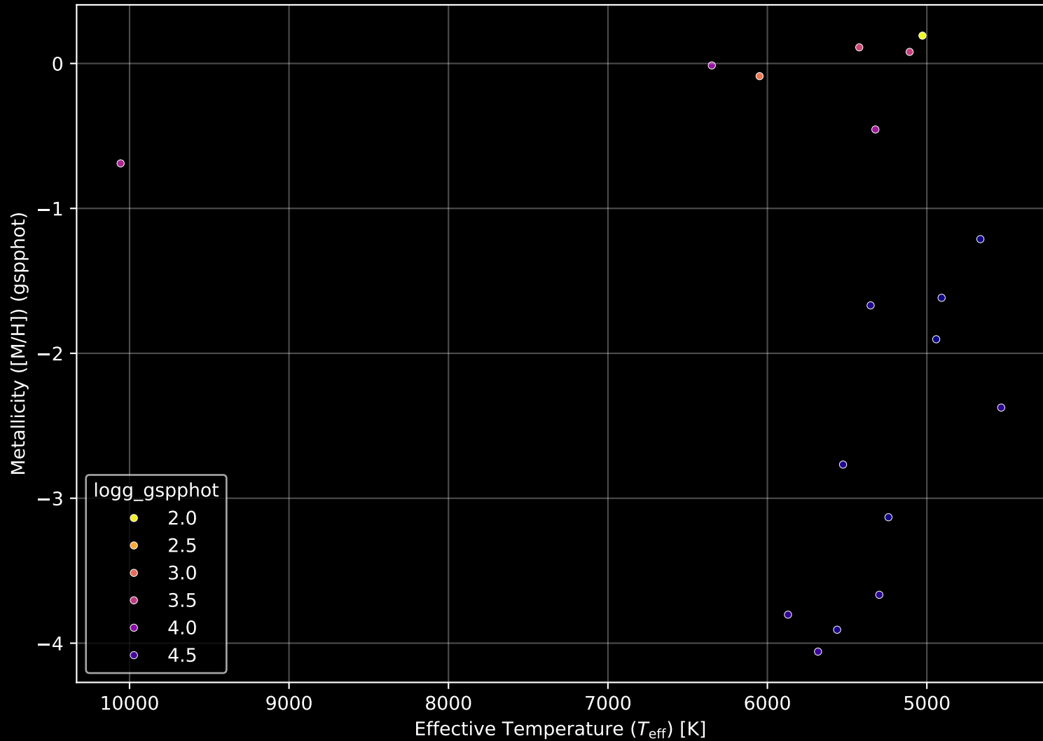
Gaia Cluster: [FSR_1171] Stellar Population Parameters (n= 18)
