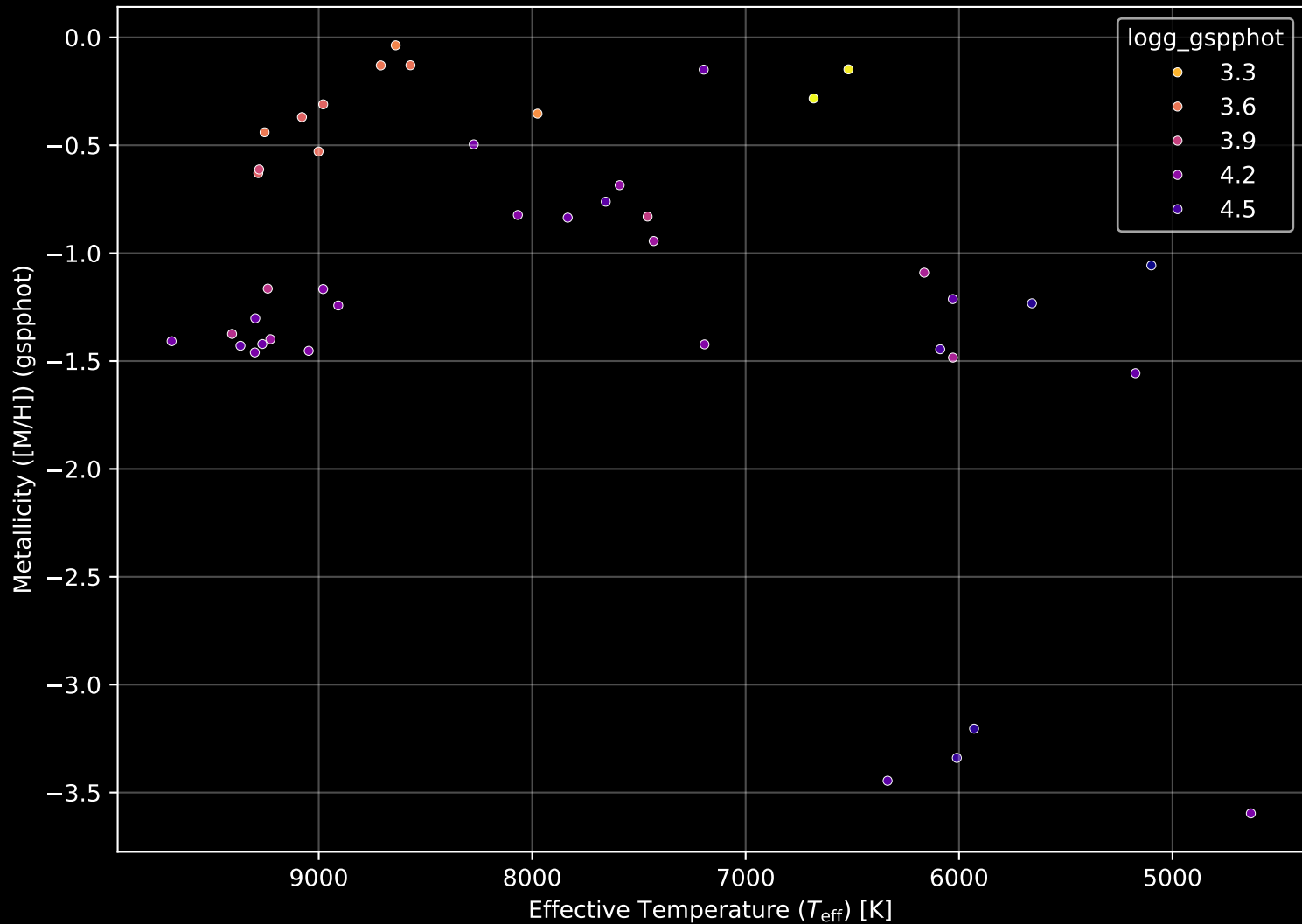
Gaia Cluster: [FSR_1484] Stellar Population Parameters (n= 43)
