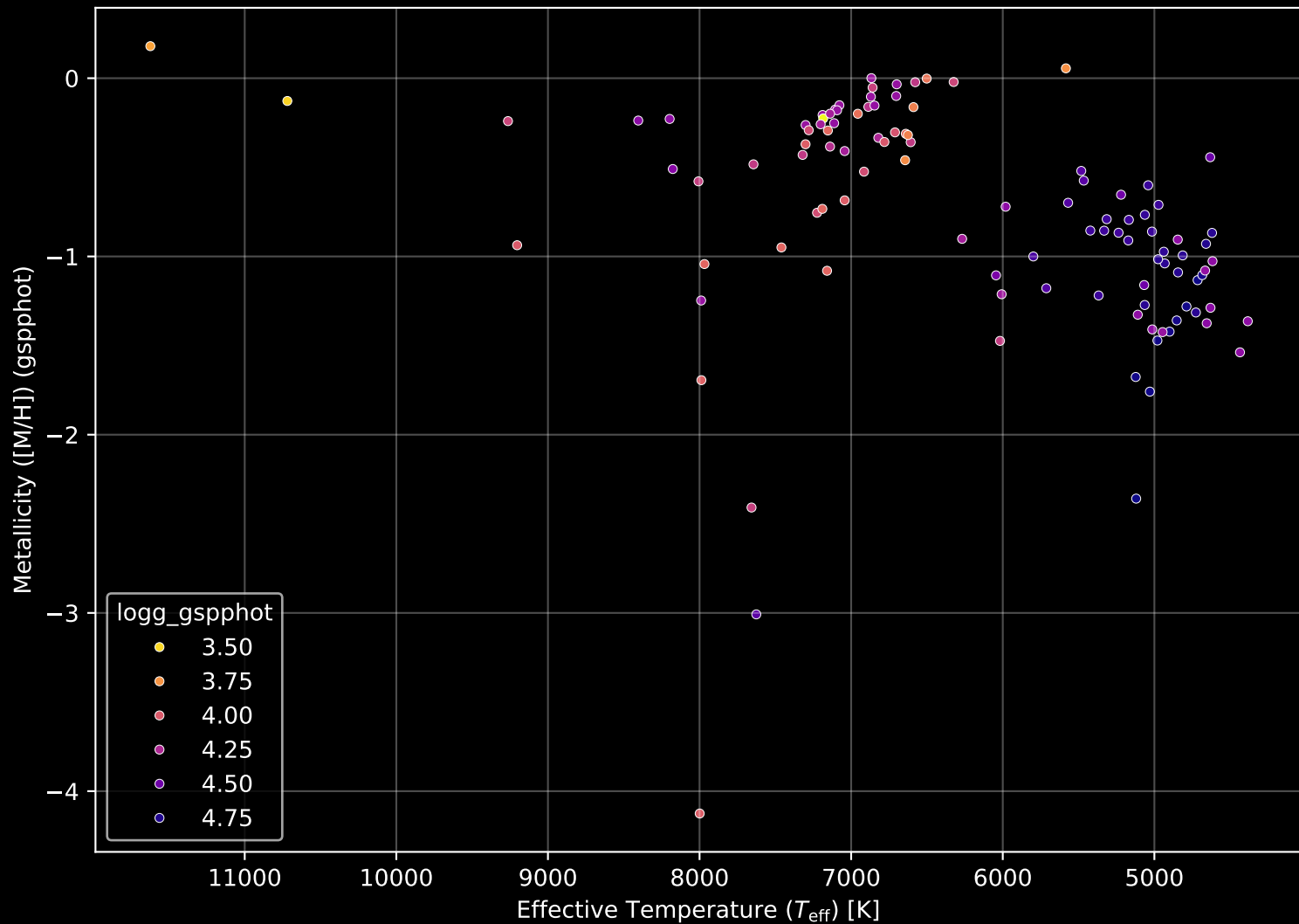
Gaia Cluster: [FSR_1723] Stellar Population Parameters (n= 108)
