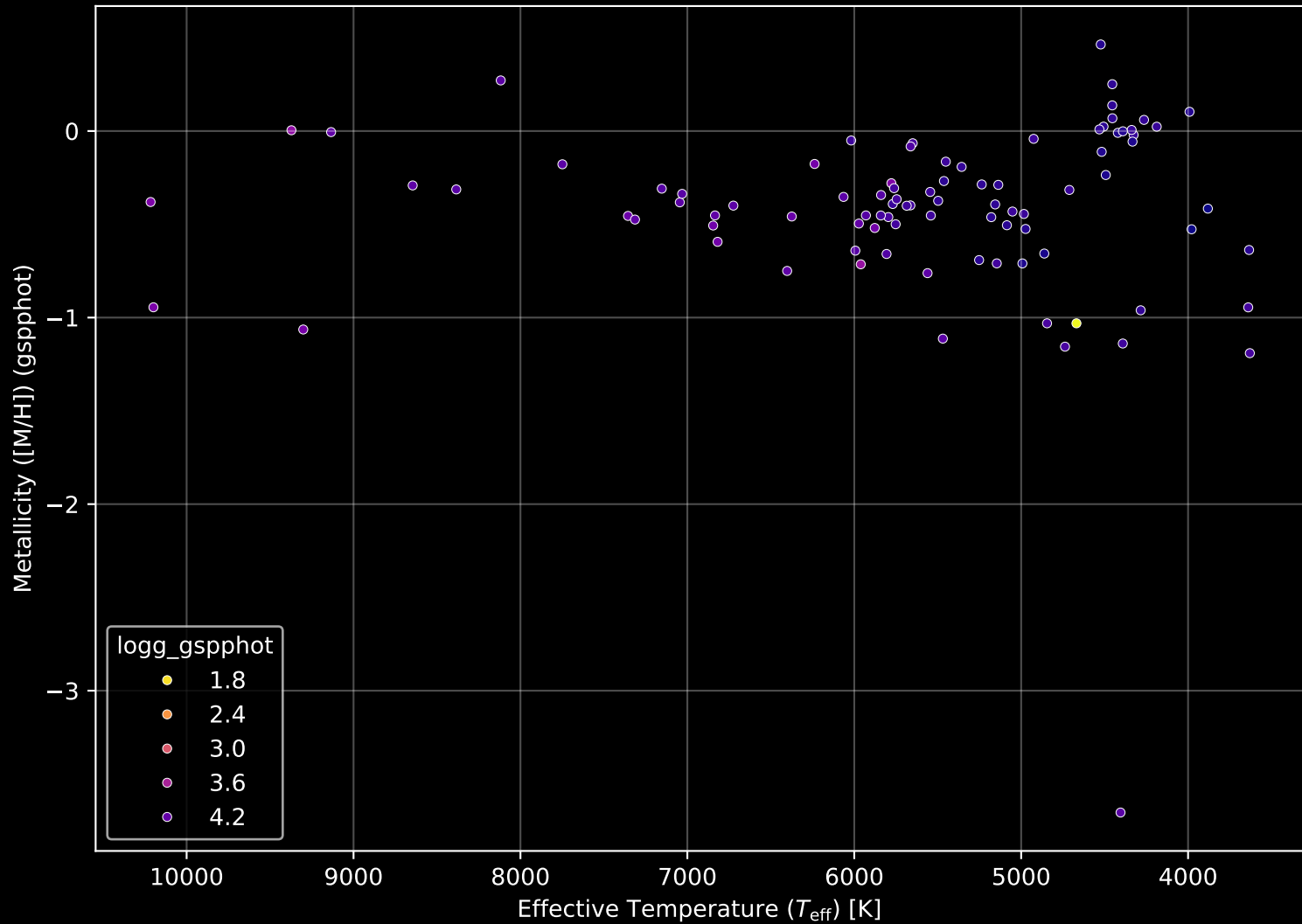
Gaia Cluster: [Ferrero_11] Stellar Population Parameters (n= 90)
