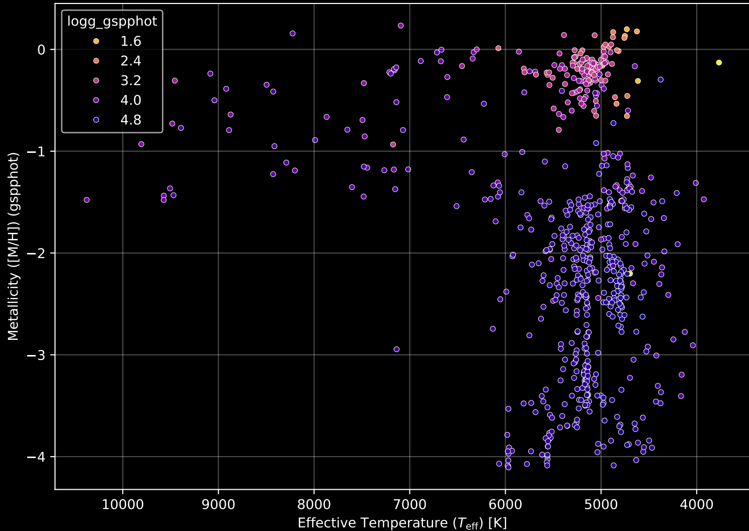
Gaia Cluster: [Gaia_1] Stellar Population Parameters (n= 663)
