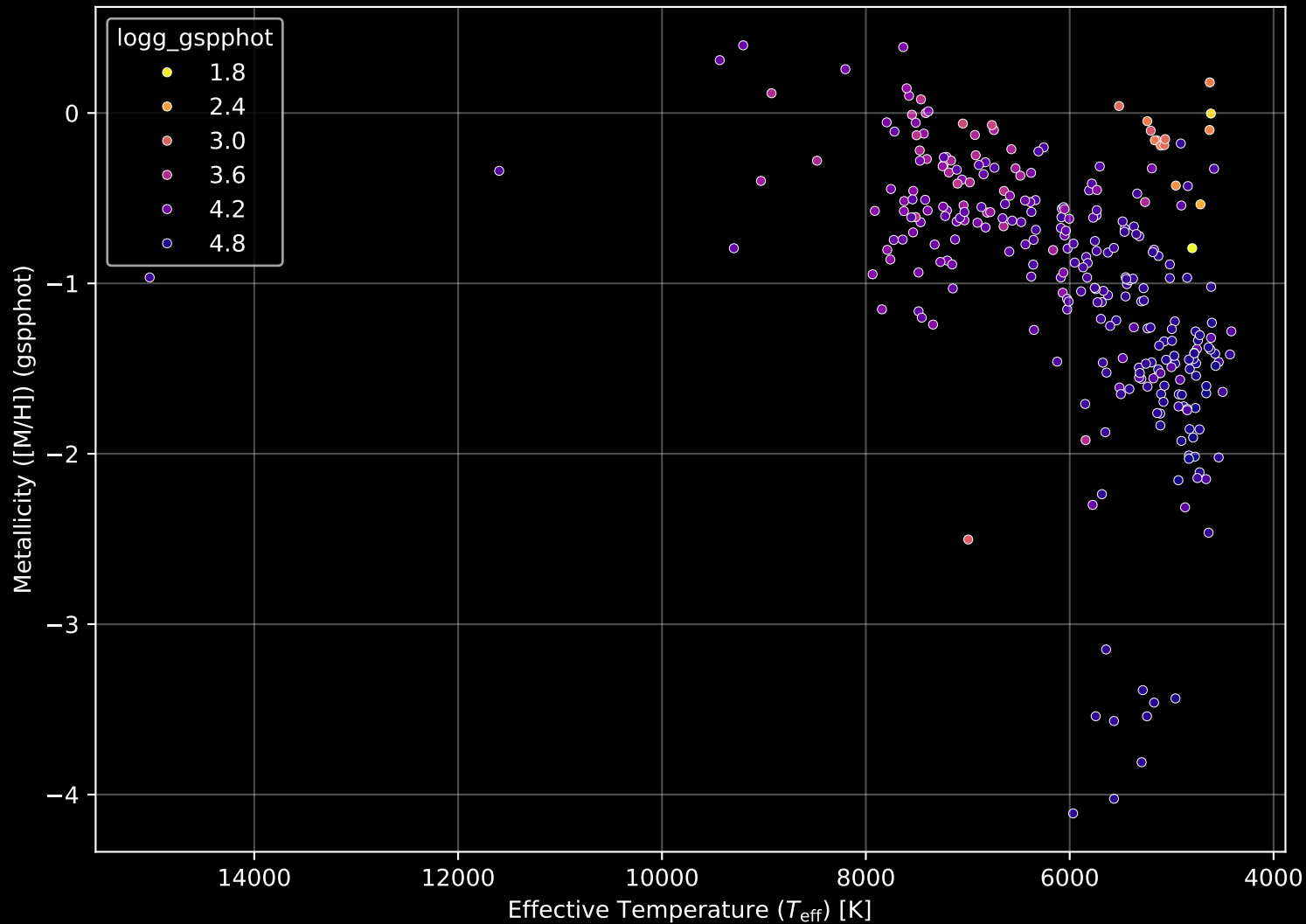
Gaia Cluster: [Gulliver_1] Stellar Population Parameters (n= 291)
