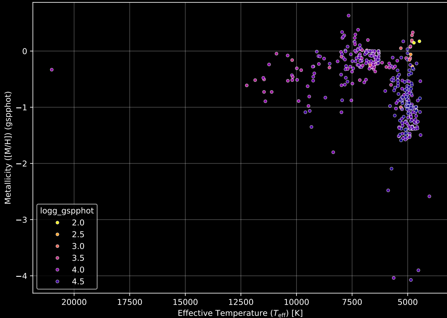
Gaia Cluster: [Gulliver_18] Stellar Population Parameters (n= 385)
