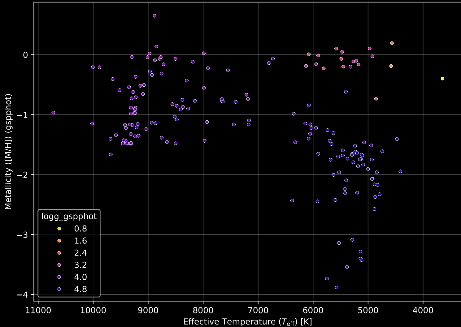
Gaia Cluster: [Gulliver_4] Stellar Population Parameters (n= 171)
