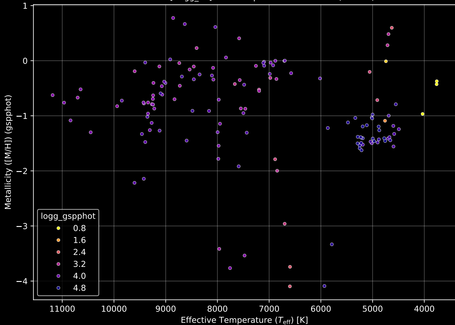
Gaia Cluster: [Hogg_17] Stellar Population Parameters (n= 142)
