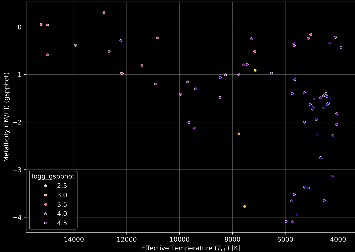
Gaia Cluster: [Ivanov_4] Stellar Population Parameters (n= 67)
