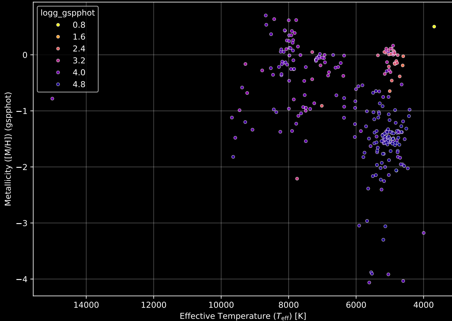
Gaia Cluster: [Juchert_13] Stellar Population Parameters (n= 279)
