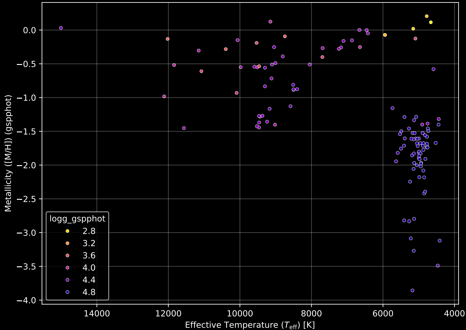
Gaia Cluster: [Juchert_20] Stellar Population Parameters (n= 124)
