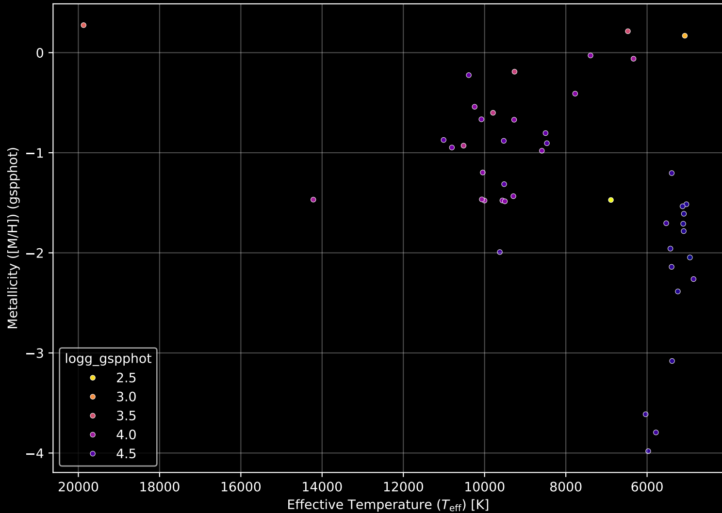
Gaia Cluster: [Juchert_9] Stellar Population Parameters (n= 45)
