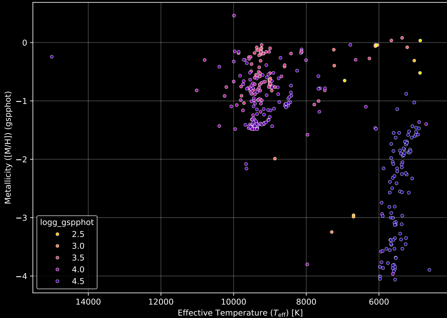
Gaia Cluster: [King_13] Stellar Population Parameters (n= 341)
