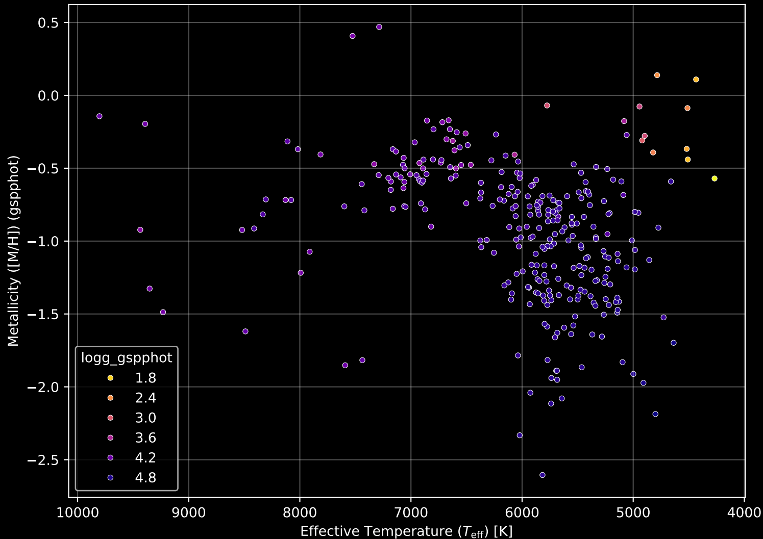
Gaia Cluster: [King_23] Stellar Population Parameters (n= 295)
