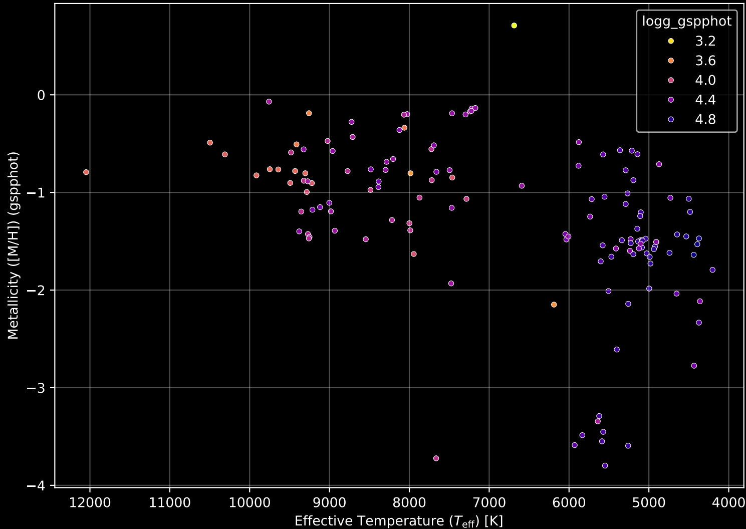
Gaia Cluster: [Koposov_36] Stellar Population Parameters (n= 140)
