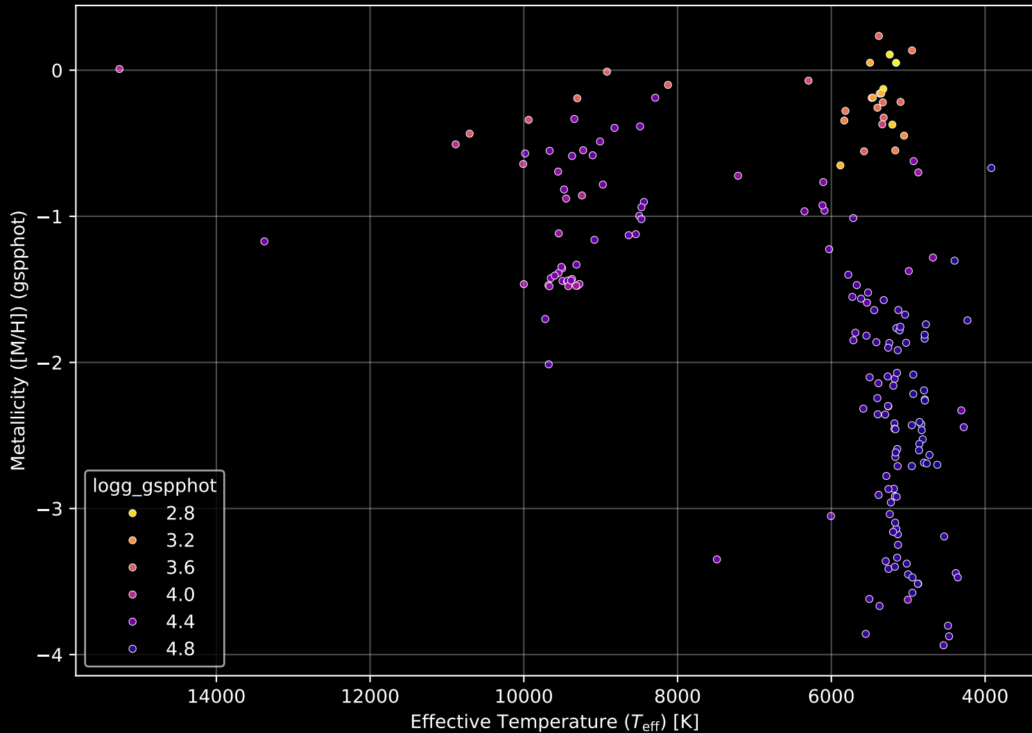
Gaia Cluster: [Koposov_63] Stellar Population Parameters (n= 186)
