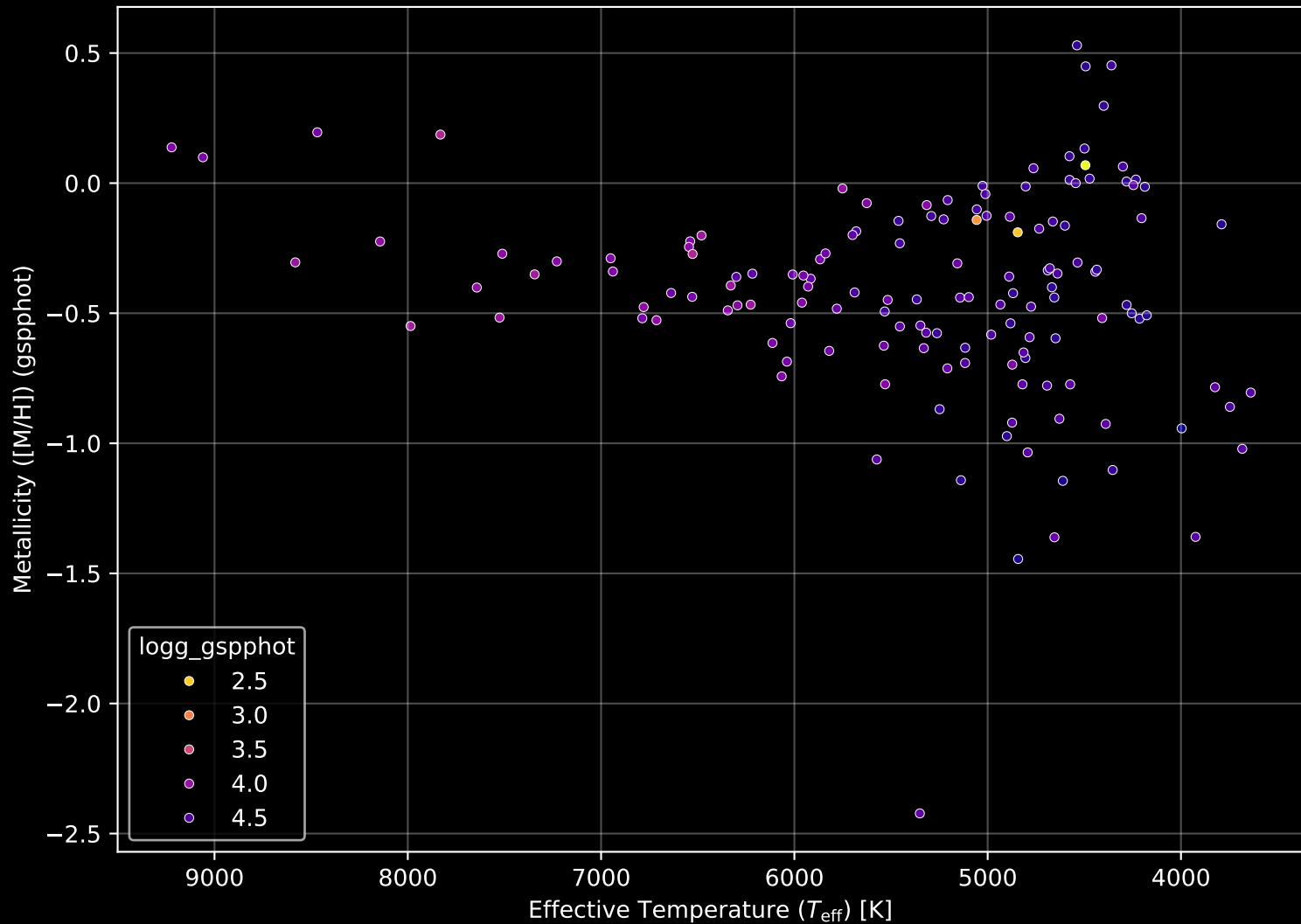
Gaia Cluster: [Loden_46] Stellar Population Parameters (n= 144)
