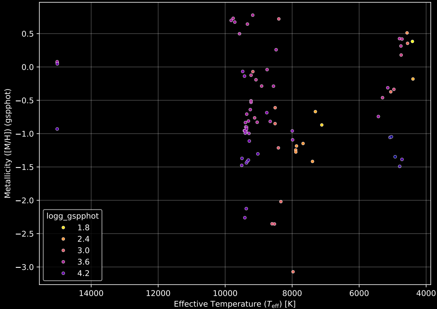
Gaia Cluster: [Lynga_3] Stellar Population Parameters (n= 81)
