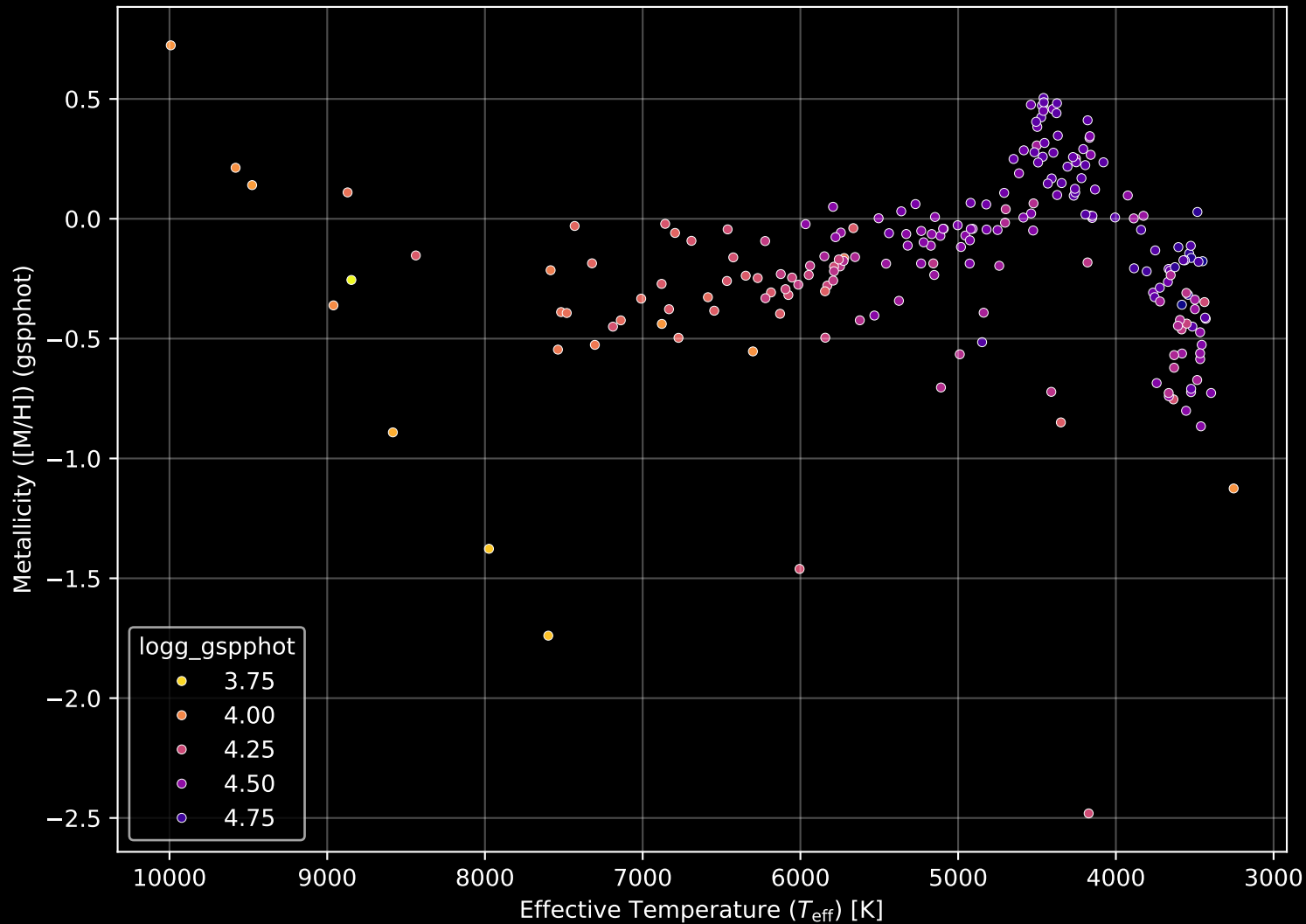
Gaia Cluster: [Mamajek_4] Stellar Population Parameters (n= 215)
