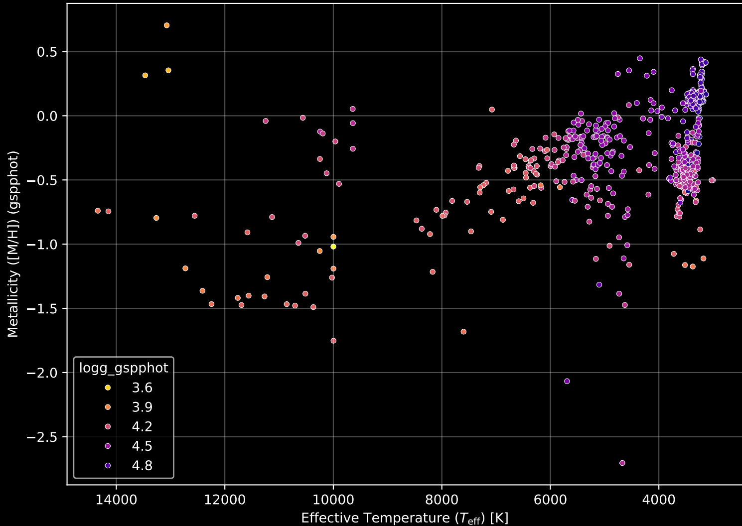
Gaia Cluster: [Melotte_20] Stellar Population Parameters (n= 657)
