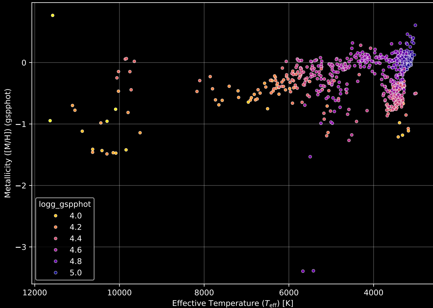
Gaia Cluster: [Melotte_22] Stellar Population Parameters (n= 947)
