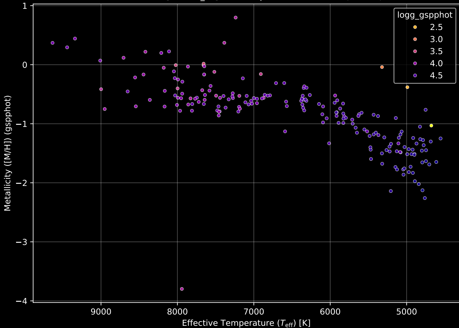
Gaia Cluster: [Melotte_72] Stellar Population Parameters (n= 194)
