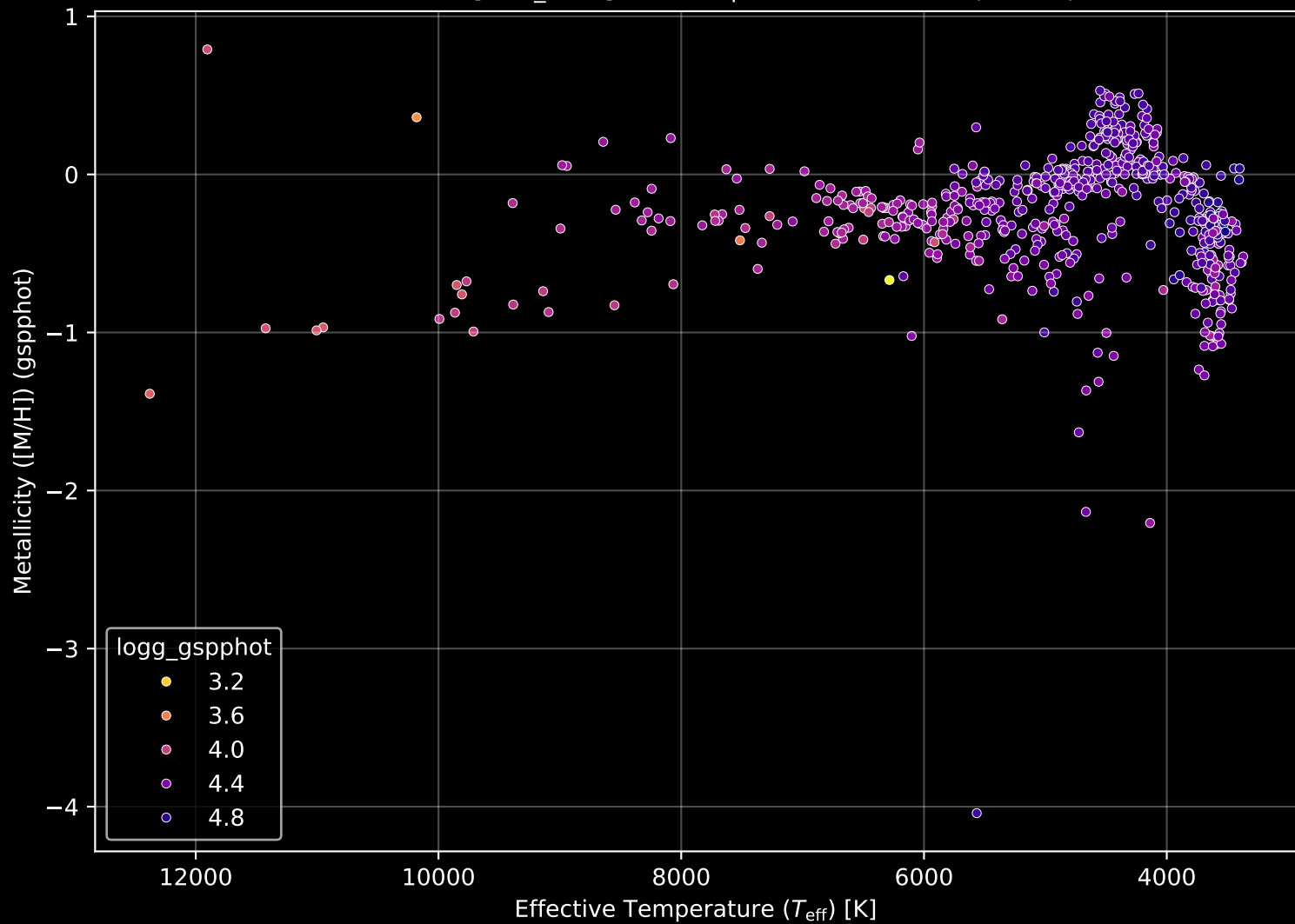
Gaia Cluster: [NGC_1039] Stellar Population Parameters (n= 607)
