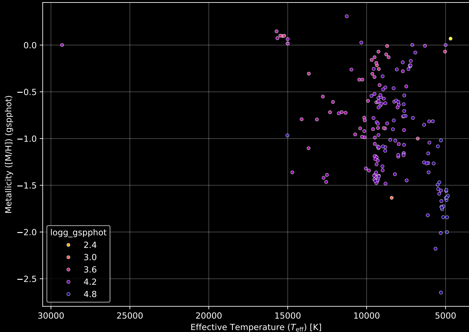
Gaia Cluster: [NGC_146] Stellar Population Parameters (n= 188)
