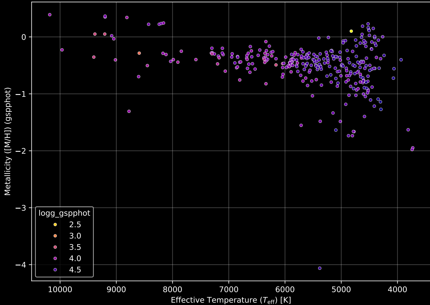
Gaia Cluster: [NGC_1528] Stellar Population Parameters (n= 303)
