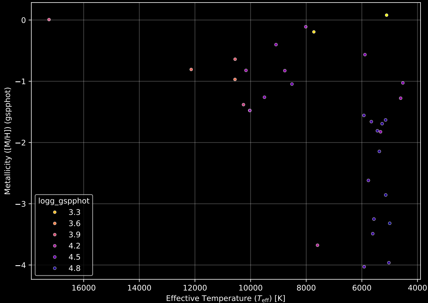
Gaia Cluster: [NGC_1624] Stellar Population Parameters (n= 33)
