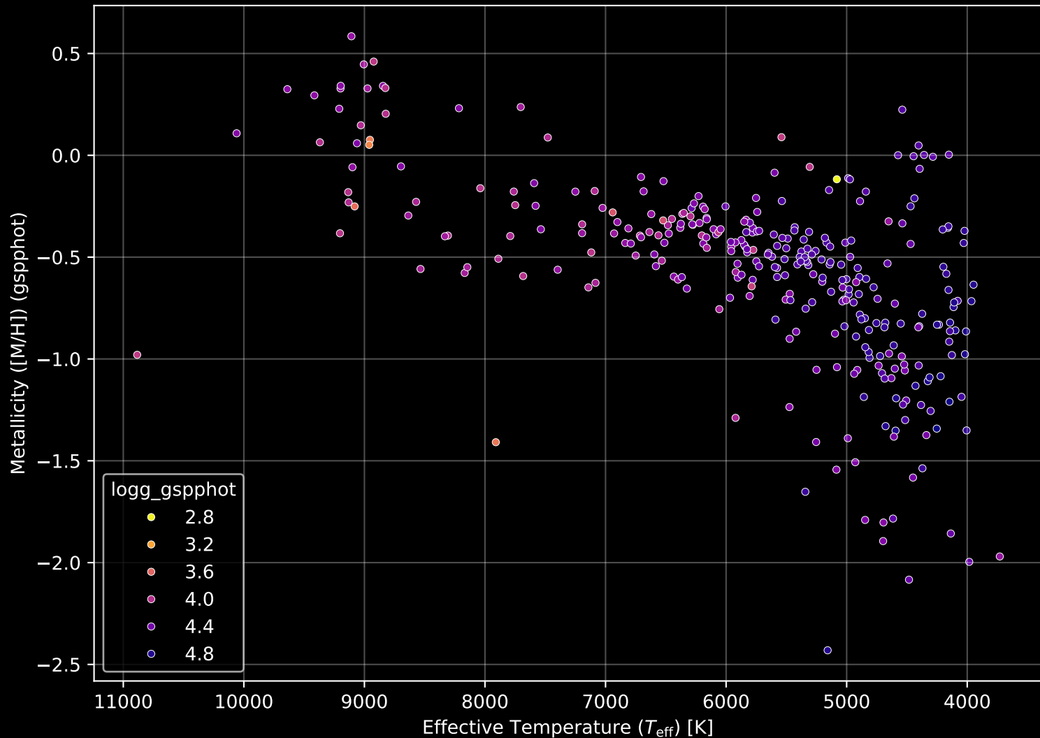
Gaia Cluster: [NGC_1664] Stellar Population Parameters (n= 320)
