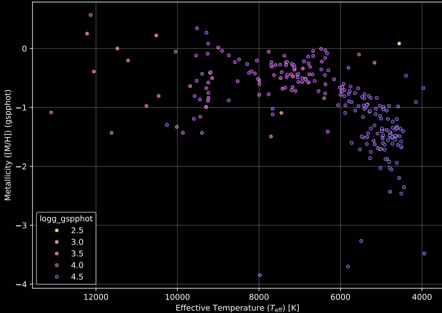
Gaia Cluster: [NGC_1778] Stellar Population Parameters (n= 243)
