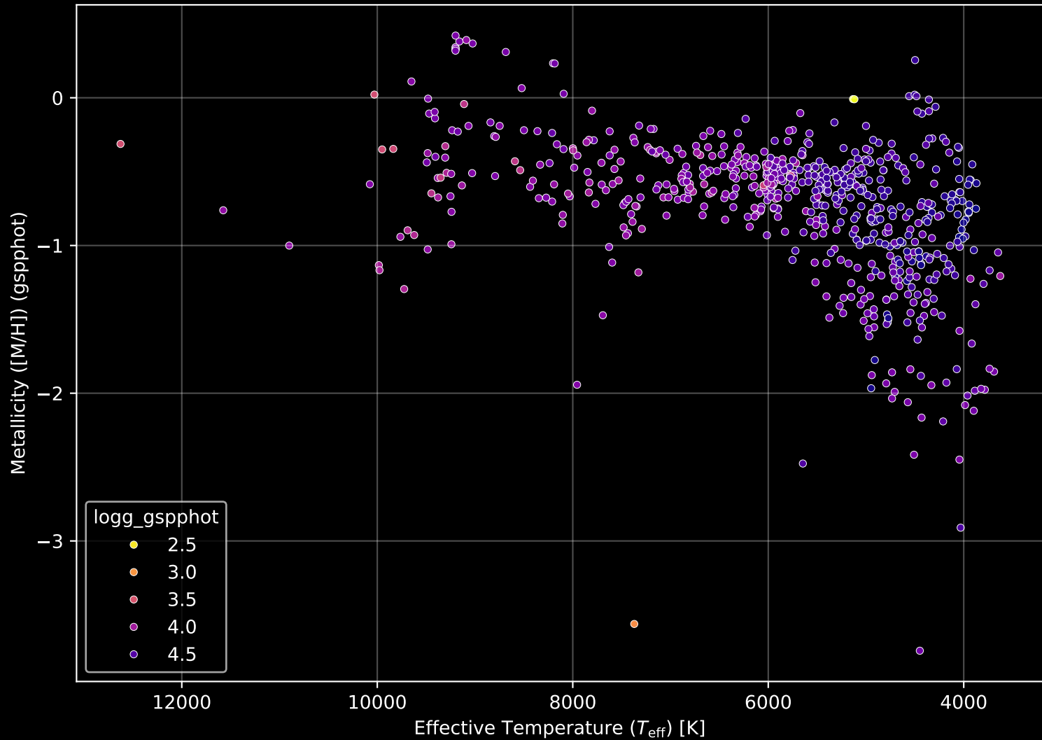
Gaia Cluster: [NGC_1912] Stellar Population Parameters (n= 668)
