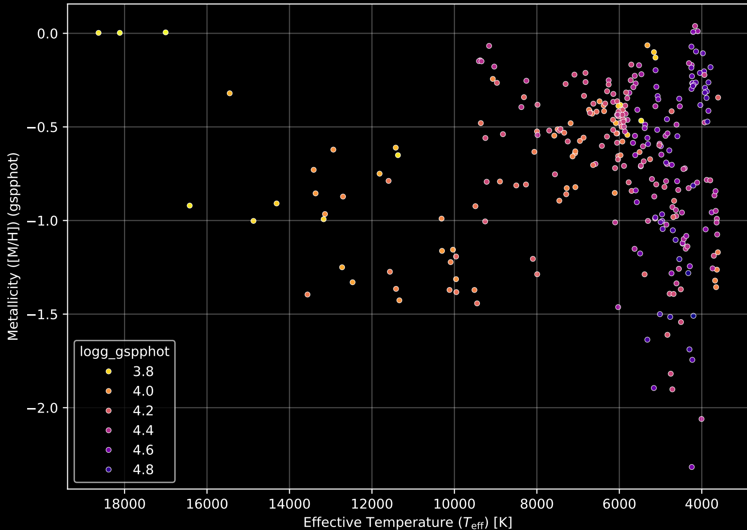
Gaia Cluster: [NGC_1960] Stellar Population Parameters (n= 296)
