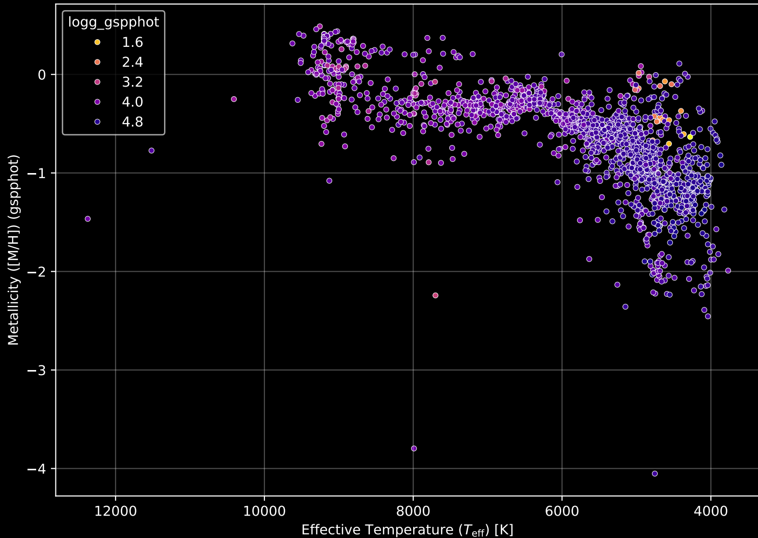
Gaia Cluster: [NGC_2099] Stellar Population Parameters (n= 1644)
