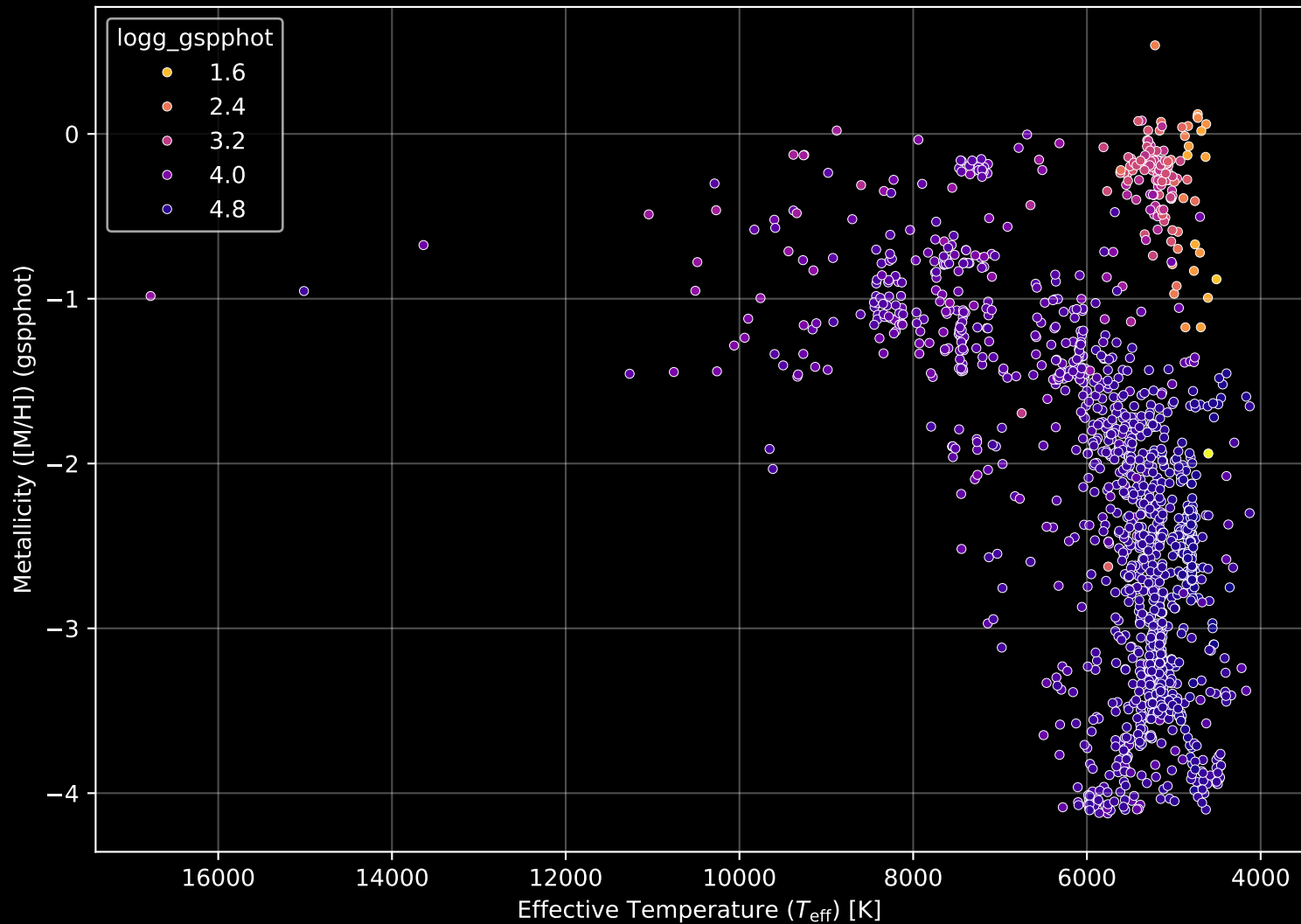
Gaia Cluster: [NGC_2158] Stellar Population Parameters (n= 1390)
